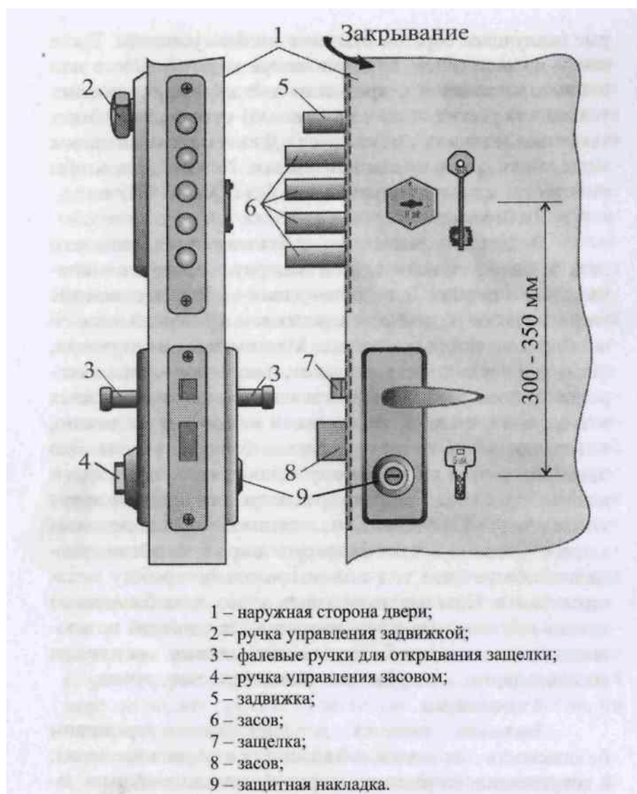
Рис. 18 - Пример оборудования двери двумя врезными замками
