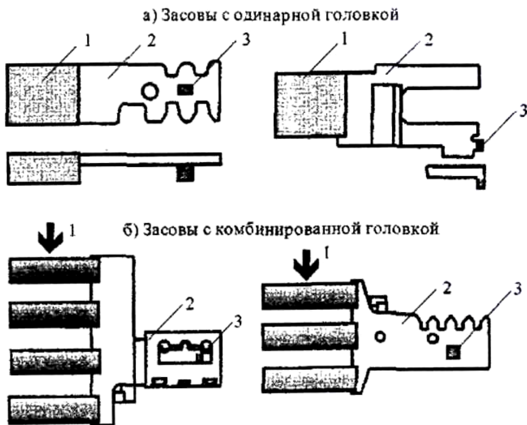
Рисунок I - Примеры и устройство засовов:
