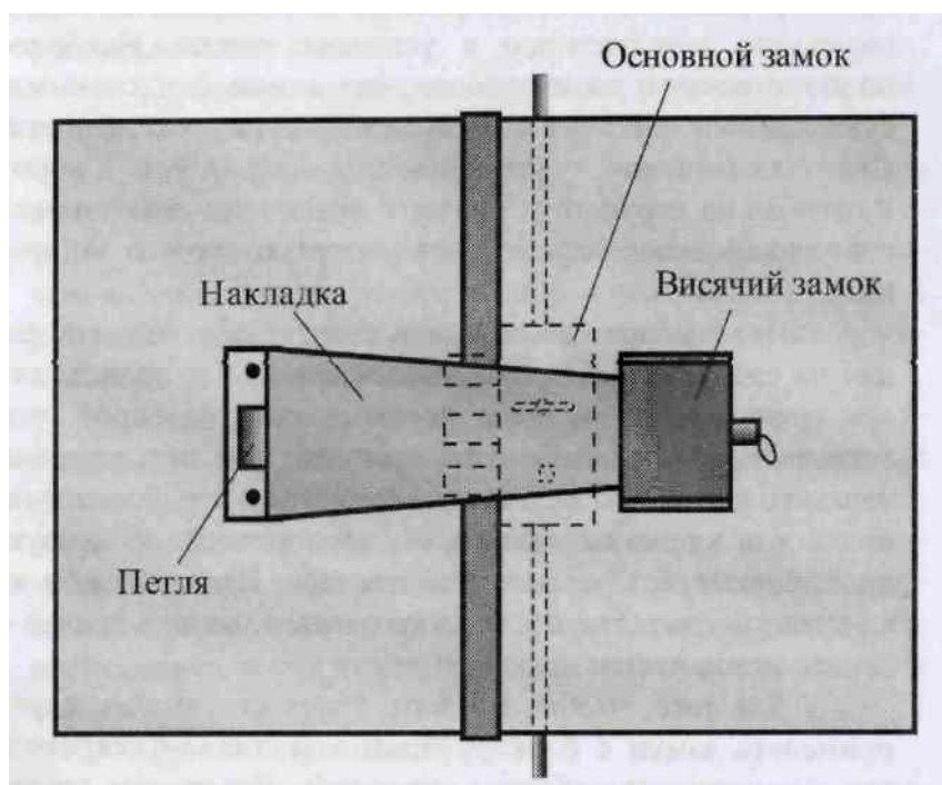
Рисунок 19 - Блокировка гаражных ворот
