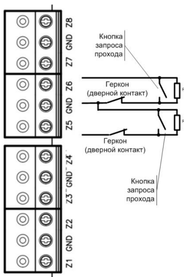
Рис.15. Подключение комбинированного шлейфа
