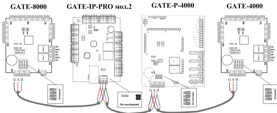
Рис.21. Контроллер Gate-IP-Pro мод.2 центральный на шине данных
