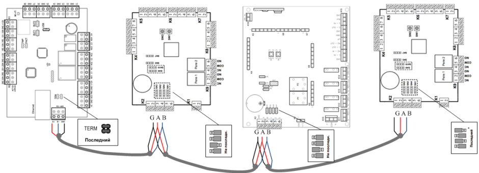
Рис.22. Контроллер Gate-IP-Pro мод.2 последний (первый) на шине данных
