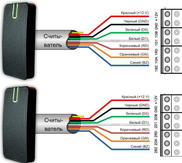
Рис.12. Подключение считывателей
