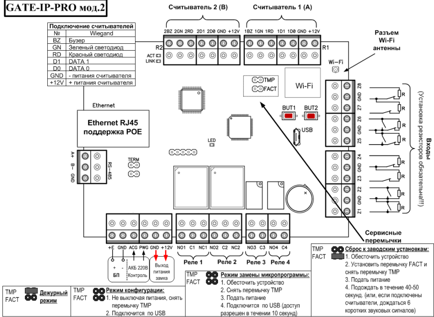
Рис. 2. Внешний вид платы контроллера
