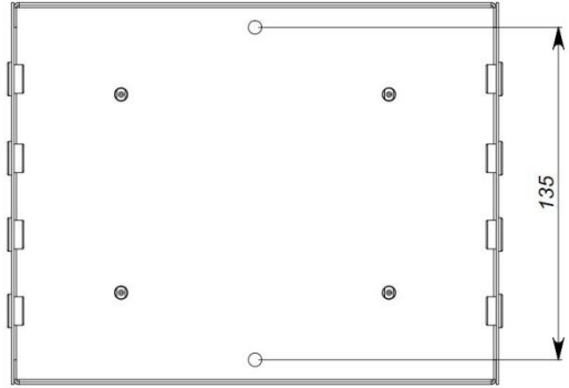
Рис 11. Разметка крепежных отверстий
