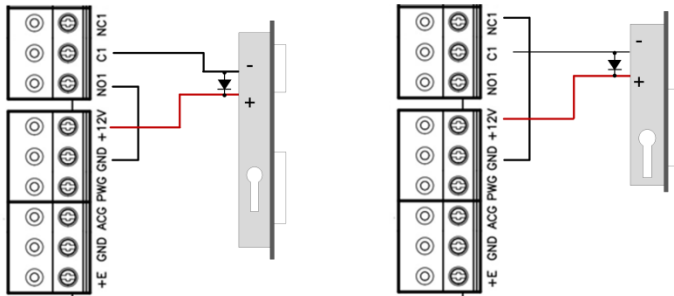
Рис.18. Подключение замков в случае использования PoE
